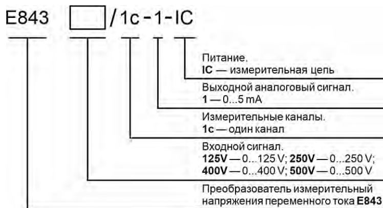
Рисунок 1 – Схема условного обозначения ИП
