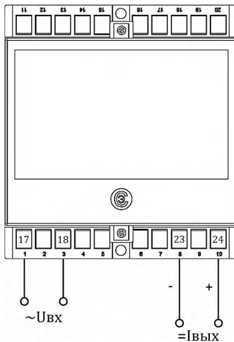
Рисунок Б.1 – Схемы электрические подключения ИП в корпусе E20
